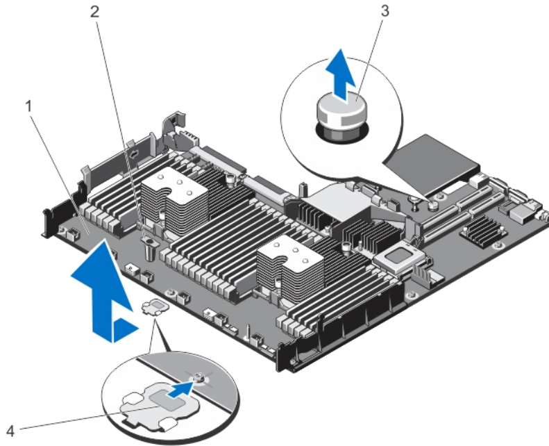
图 44: 卸下和安装系统板
