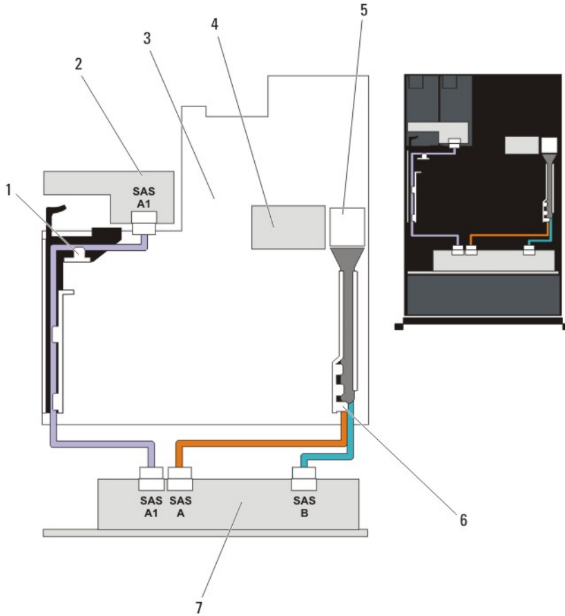
图 42: 布线图—可选 2.5 英寸 (x2) 硬盘驱动器背板（背面）
