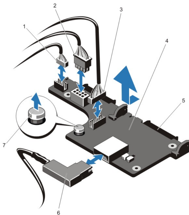
图 41: 卸下和安装可选 2.5 英寸 (x2) 硬盘驱动器背板
