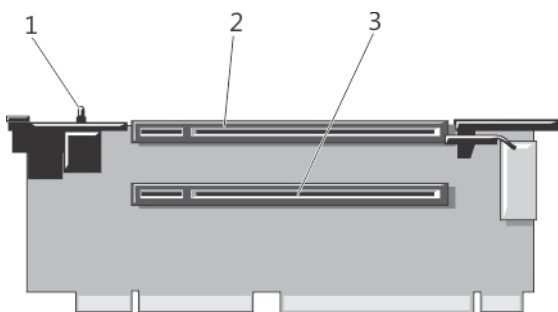
图 27: 识别扩充卡提升板 2 上的连接器
