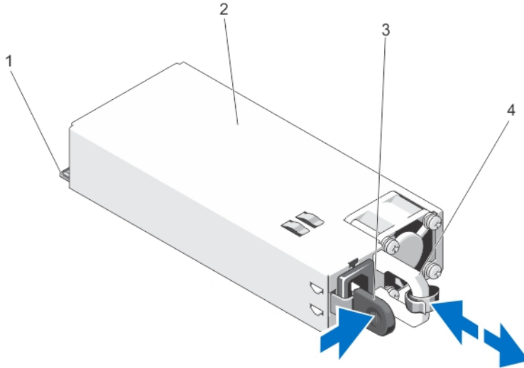
图 36: 卸下和安装交流电源设备
