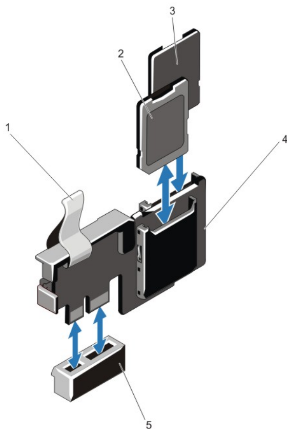
图 30: 卸下和安装内部双 SD 模块
