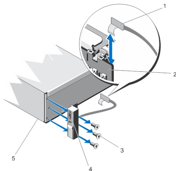
图 43: 卸下和安装 I/O 面板
