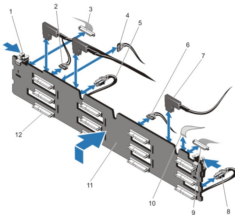
图 39: 卸下和安装 3.5 英寸 (x12) SAS 背板
