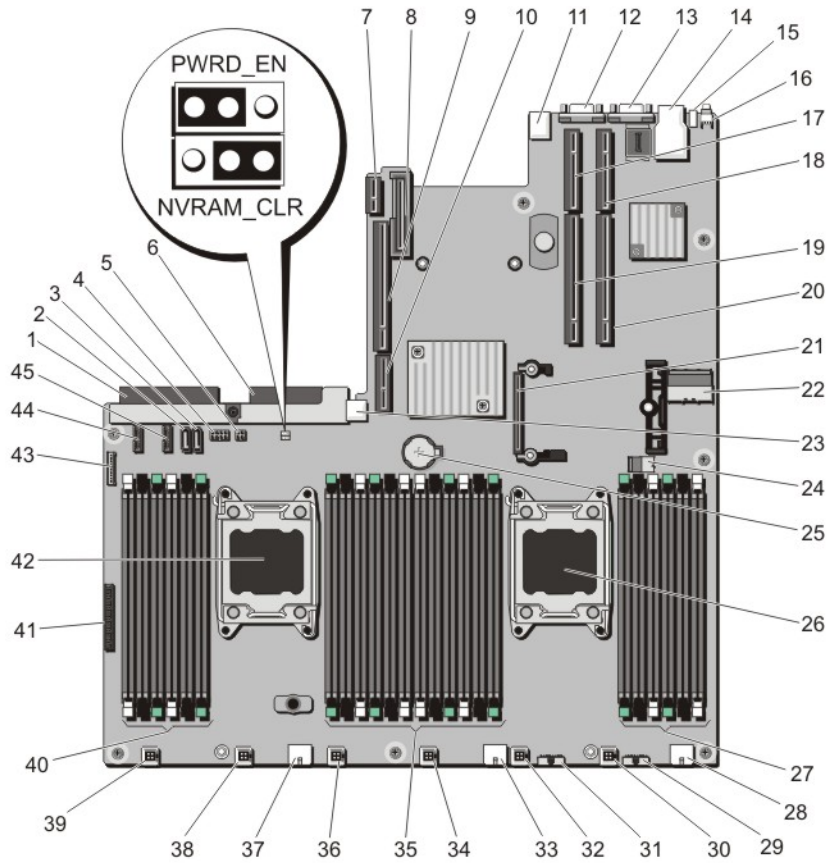
图 45: 系统板跳线和连接器
