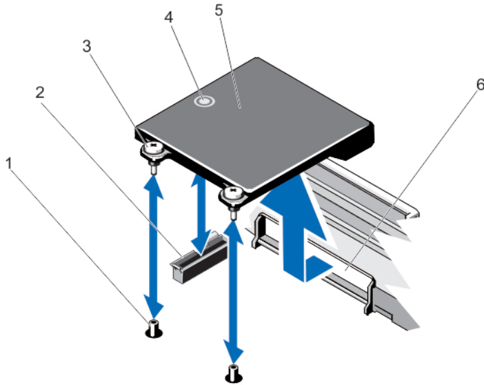
图 32: 卸下和安装网络子卡
