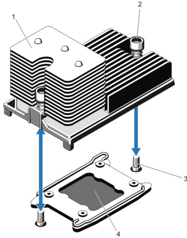
图 33: 卸下和安装处理器散热器
